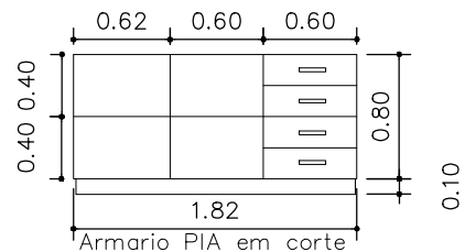
Armario PIA em corte
